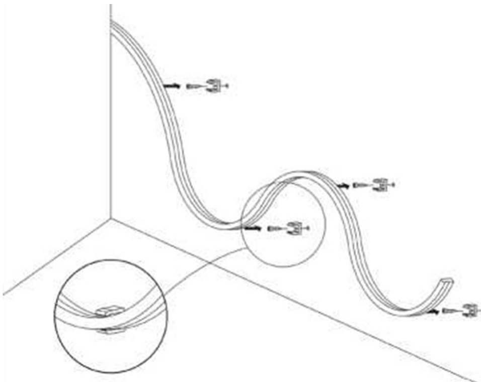
КРИВОЛИНЕЙНАЯ УСТАНОВКА НА СКОБЫ
