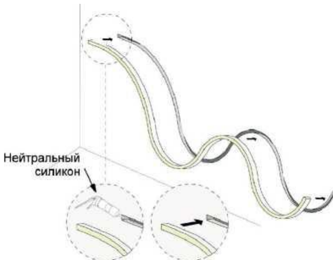
КРИВОЛИНЕЙНАЯ УСТАНОВКА В ПАЗ
