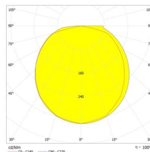
Рисунок 3 – Световое распределение.
