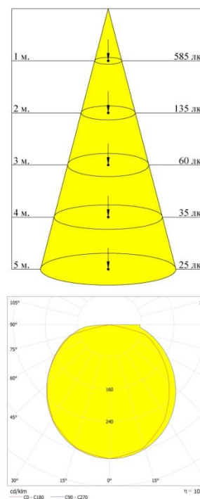
Рисунок 3 – Световое распределение.
