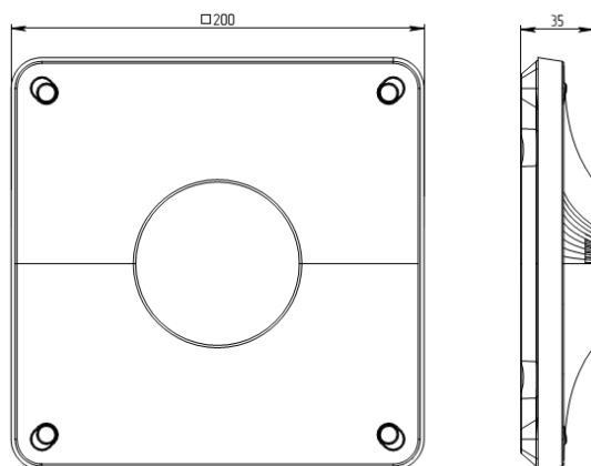
Рисунок 2 – Габаритный чертеж.
