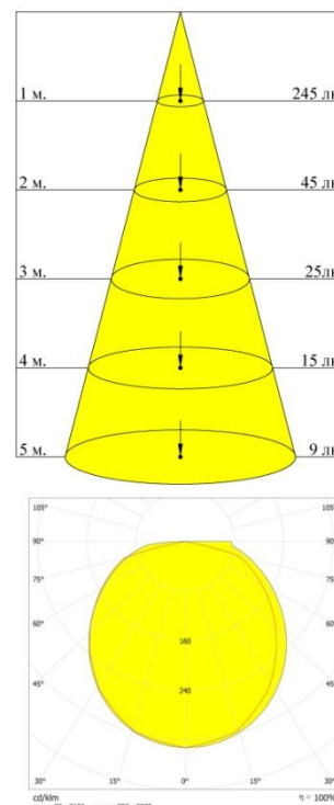
Рисунок 3 – Световое распределение.
