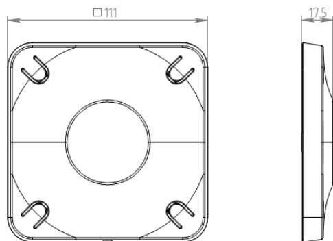
Рисунок 2 – Габаритный чертеж.
