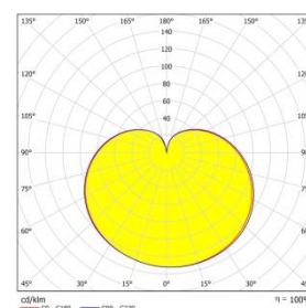
Рисунок 2 – Световое распределение лампы E27 A60 7W.
