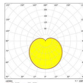
Рисунок 2 – Световое распределение лампы E27 G45 5W.
