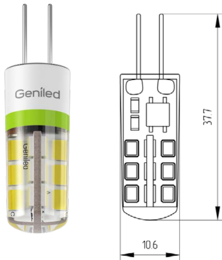
Рисунок 1 – Внешний вид и чертёж.
